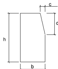
Rys. 1. Wymiarowanie krawężnika typ U
